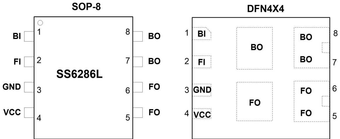
图 1. 顶视图
