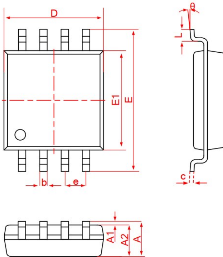
图 20: SOP-8 封装信息
